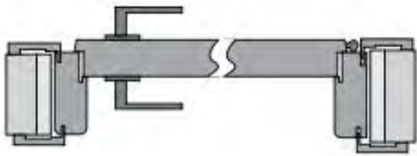
Раздвижная одностворчатая дверь снаружи стены
