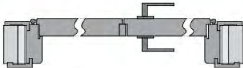
Раздвижная двустворчатая дверь снаружи стены
